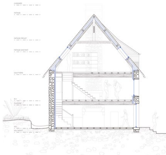
↘ Réhabilitation d'un corps de ferme. Coupe, 2023 (étude en cours)
