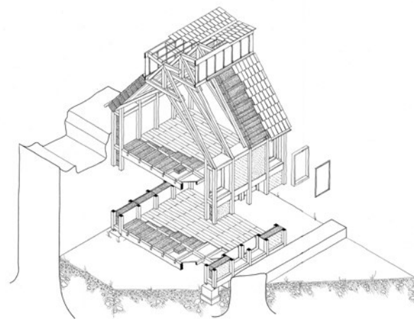
↘ Récit prospectif en monument classé, Château de la Hunaudaye (22), axonométrie, 2024
